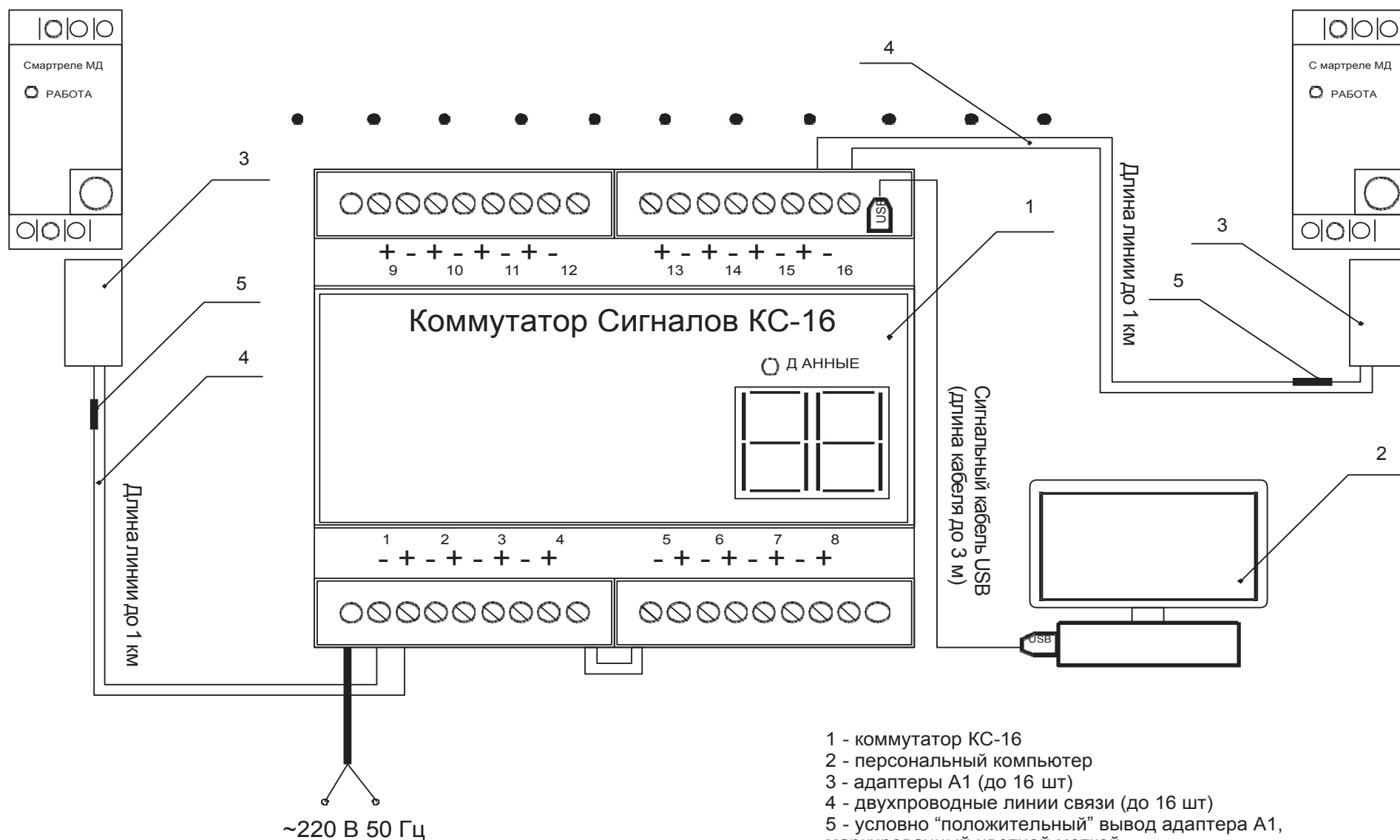
Рисунок 17 – подключение монитора двигателя МД-4М к ПК при помощи коммутатора сигналов КС-16 (система «СИРИУС»)
