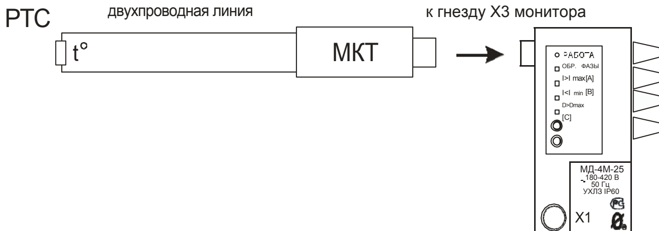
Рисунок 28 – подключение модуля контроля температуры
