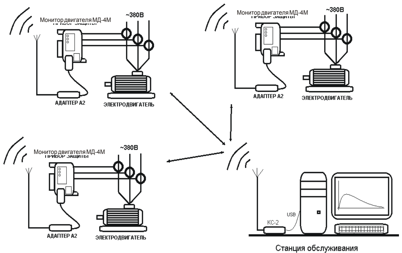
Рисунок 27 – схема организации связи в сети беспроводного доступа
